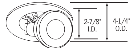
CTR320-(P, B, BC) Retractable Pull Down
