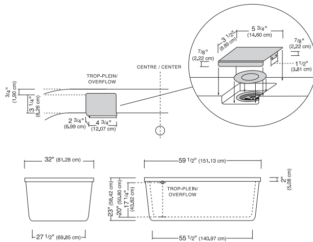
TAO 3260 avec jupe contour et trop plein Ultim-O / TAO 3260 with skirt and Ultim-O overflow
